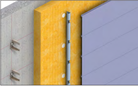
Abb. 11 Hinterlüftete Fassade waagrecht auf Betonwand mit Dämmung (PHMW1)
