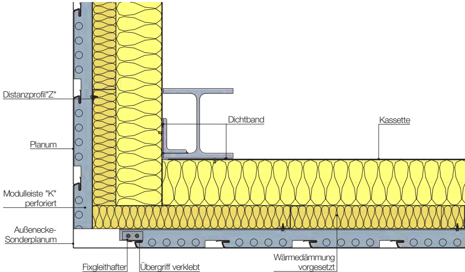
Abb. 42 Eckausbildung bei lotrechter Planum-Fassade (PHKS 102)
