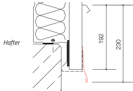
Abb. 59 Fußprofil
