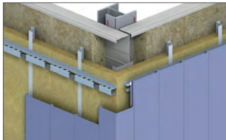
Abb. 17 Außenecke mit Sonderplanum – Planum senkrecht auf Kassetten-Innenschale (PHKS 102)
