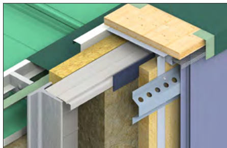
Abb. 51 Fixpunktprofil 'K' perforiert für senkrechte Verlegung auf waagrechtter Kasette (PHKSF354)
