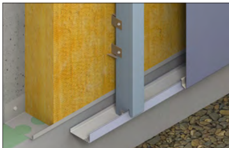
Abb. 46 Unterer Fassadenabschluss Planum VO-Ausführung
