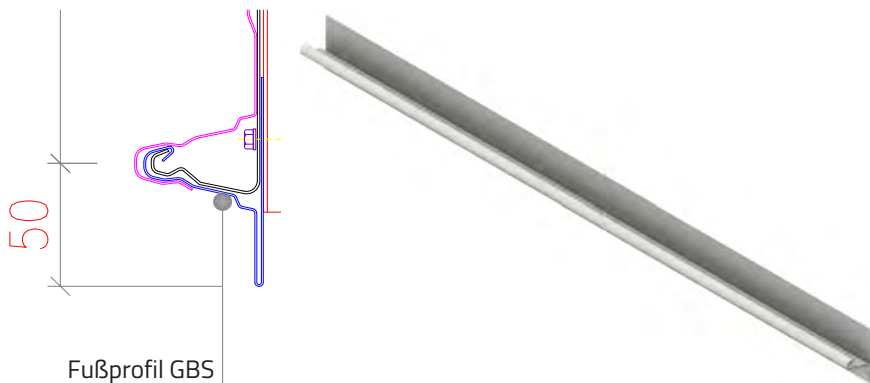
Abb. 66 Fußprofil (siehe Details Kapitel 6./Materialliste), Schnitt des Fußprofils
