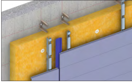
Abb. 13 Hinterlüftete Fassade waagrecht mit Schattenfuge auf Betonwand und Dämmung (PHMW001)
