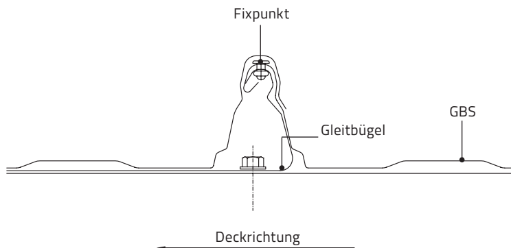
Abb. 67 Fixpunktausbildung
