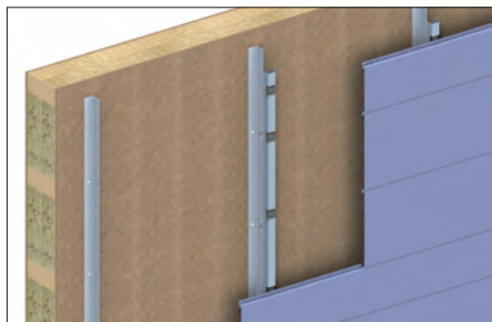
Abb. 31 Hinterlüftete Fassade waagrecht mit Ausgleichswinkel auf gedämmter Holzriegelwand (PHHW1)
