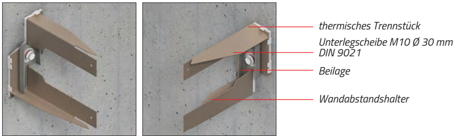
Abb. 20 Wandabstandshalter Ansicht rechts und Ansicht links mit Unterlegscheibe \varnothing 30 mm, Zulassungsnummer: Z-14.1-447
