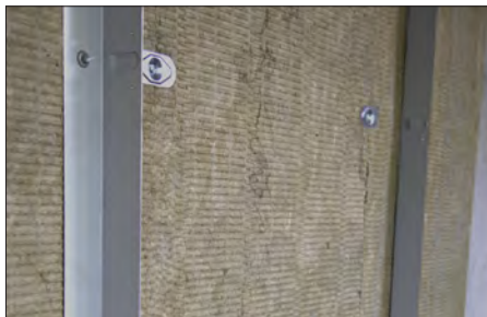
Abb. 23 Ausgleichswinkel auf Kasette mit vorgesetzter Wärmedämmung
