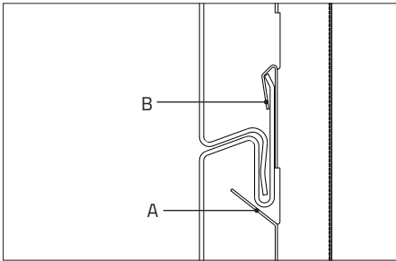
Abb. 38 Sicherung gegen Aushängen
