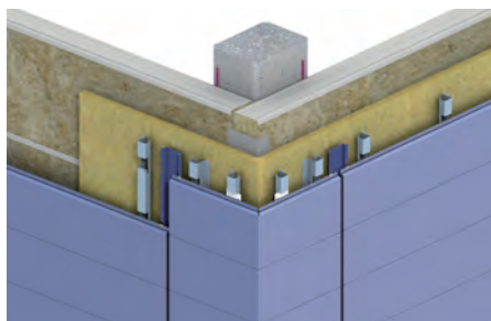
Abb. 41 Planum-Eckelement
