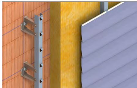
Abb. 56 Hinterlüftete Fassade waagrecht auf Mauerwerk mit Dämmung (SHMW1)
