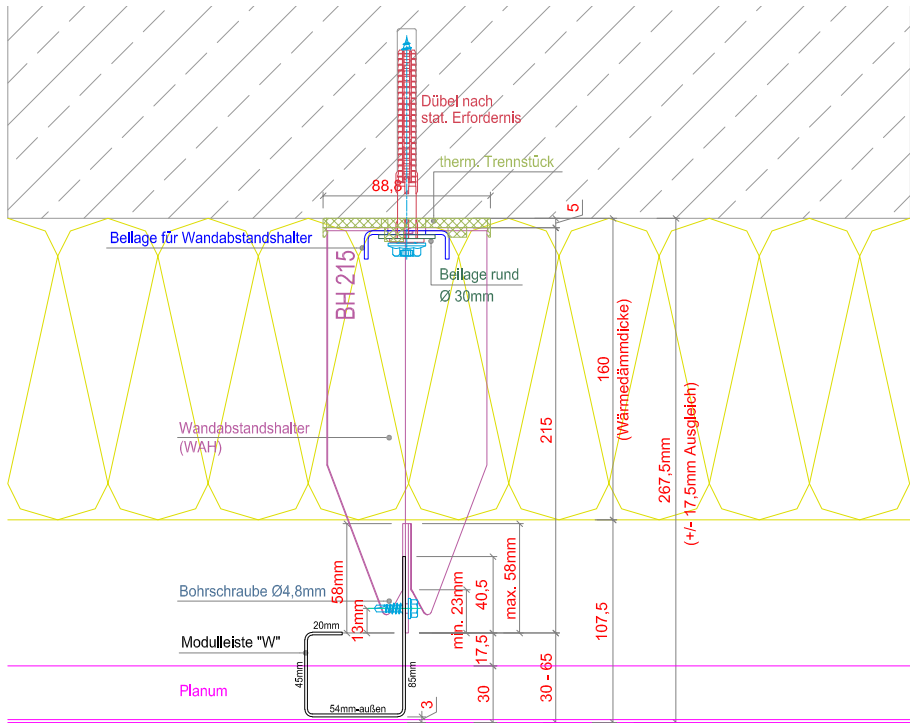
Abb. 07 Planum mit Wandabstandshalter
