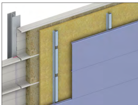
Abb. 75 Hinterlüftete Fassade waagrecht auf Kassetten-Innenschale mit vorgesetzter Dämmung (PHKW2)
