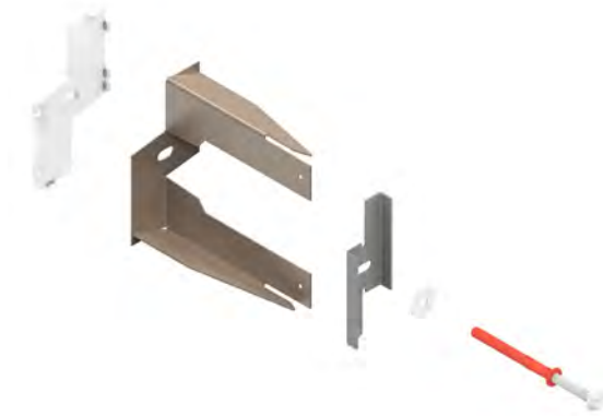
Abb. 22 Wandabstandshalter (Explosionszeichnung)
