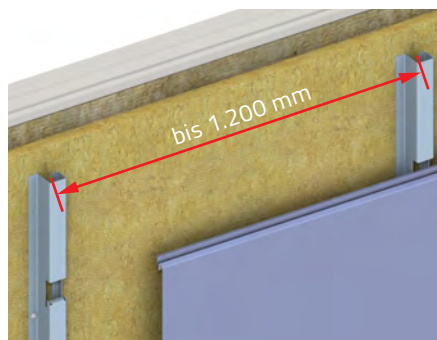
Abb. 74 Hinterlüftete Fassade waagrecht mit thermischer Trennung auf den Kassetten-Außengurten
