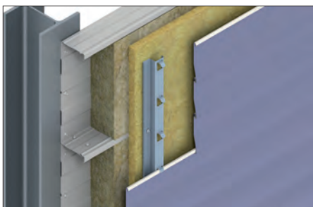
Abb. 57 Hinterlüftete Fassade waagrecht auf Kassetten-Innenschale mit vorgesetzter Dämmung (SHKW2)
