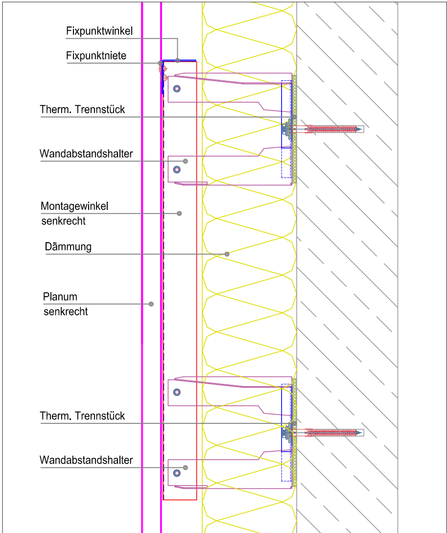
Abb. 50 Querschnitt Fixpunktausbildung Planum senkrecht
