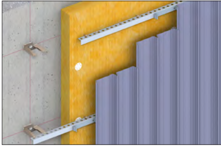
Abb. 64 Hinterlüftete Fassade senkrecht mit perforierte Montagewinkel auf Kassetten-Innenschale (GFHMS1)
