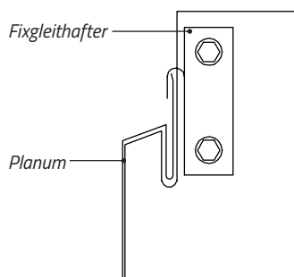
Abb. 36 Ausführung des Fixgleithafters bei waagrechtter Verlegung
