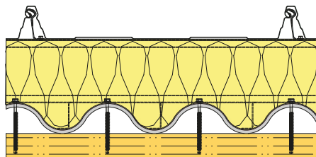
Ausführung II (gedämmt) mit Domitec-Oberschale
