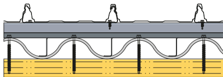
Ausführung I (ungedämmt) mit GBS-Oberschale
