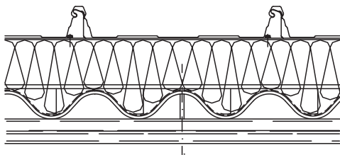
Ausführung II (gedämmt) mit Domitec®-Außenhaut
