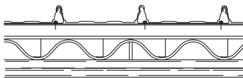
Ausführung I (ungedämmt) mit GBS®-Außenhaut
