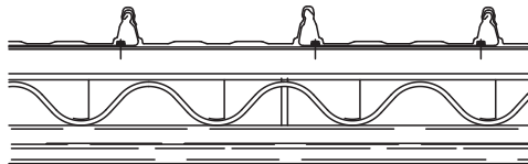
Ausführung I (ungedämmt) mit GBS-Außenhaut
